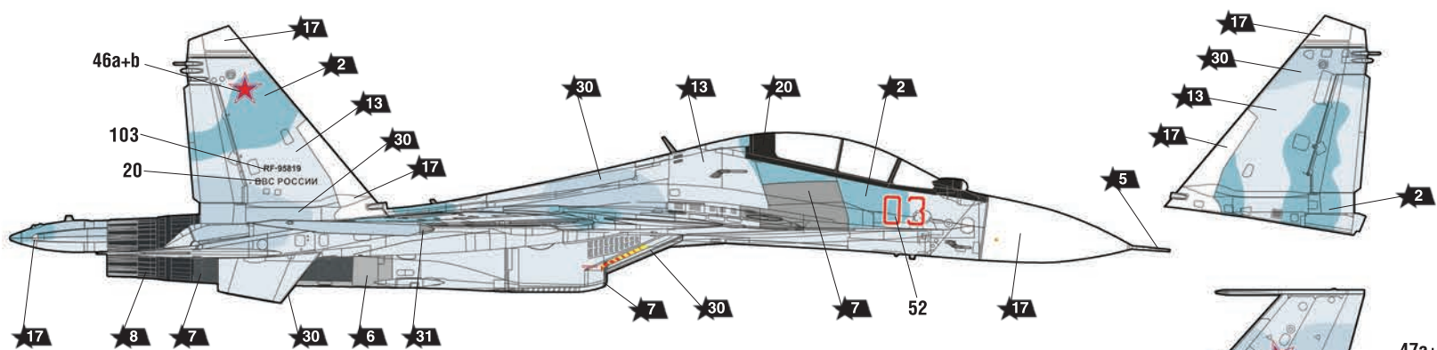
2 Су-30СМ из состава группы ВКС России в Сирии, авиабаза Хмеймим, декабрь 2017 года. Su-30SM from the Russian air force group in Syria, Hmeimim airbase, December 2017.
