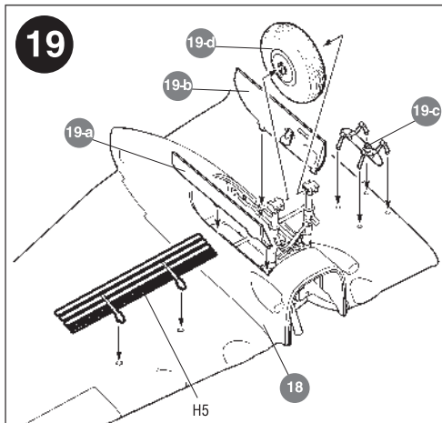
19 ДЛЯ 1 ВАРИАНТА СБОРКИ FOR ASSEMBLING VERSION 1
