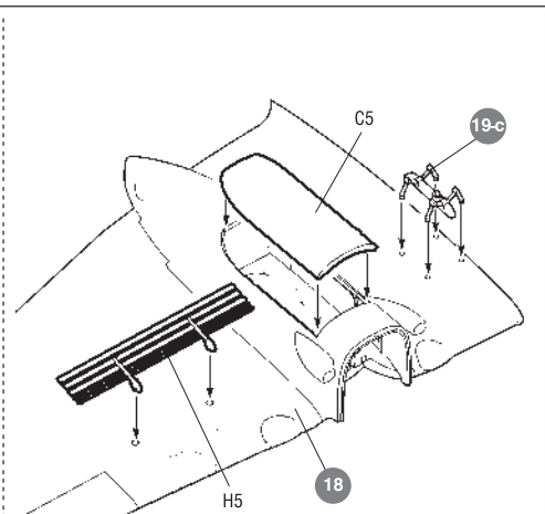
ДЛЯ 2 ВАРИАНТА СБОРКИ FOR ASSEMBLING VERSION 2
