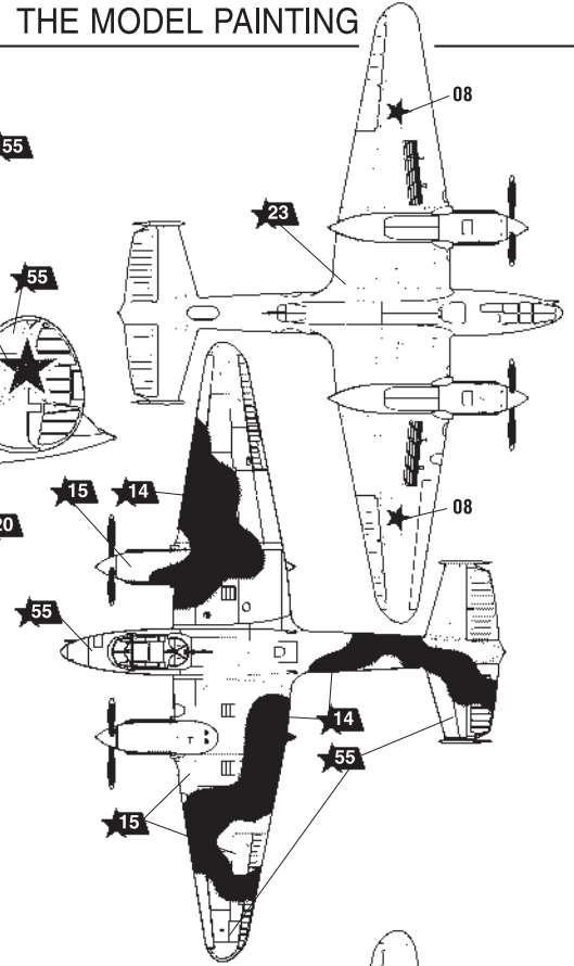
1 Пе-2 командира 12-го Гв. пикирующего Бомбардировочного Таллинского Краснознаменного ордена Ушакова Авиаполка ВВС КБФ дважды Героя Советского Союза подполковника В.И.Ракова. Лето 1944 г. 12th Guards Dive Bomber Aviation Regiment, 1944
