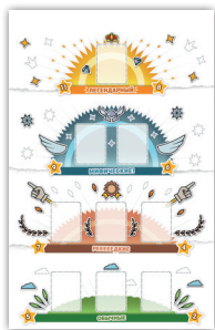
Планшет редкости
