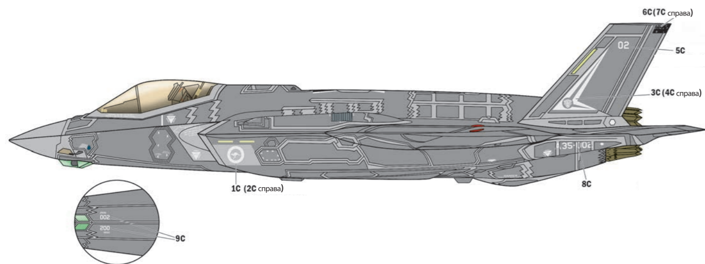
Вариант C – Королевские ВВС Австралии, 61-я испытательная эскадрилья истребителей, Вильямтаун, Австралия 2016.
