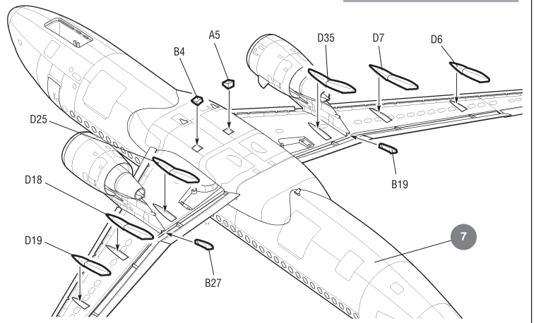
ВАРИАНТ СБОРКИ 3 ASSEMBLING VERSION 3
