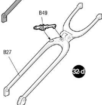
2 ВАРИАНТ СБОРКИ ASSEMBLING VERSION 2
